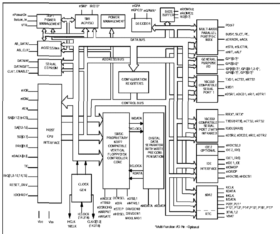
FDC37C93xAPM BLOCK DIAGRAM
