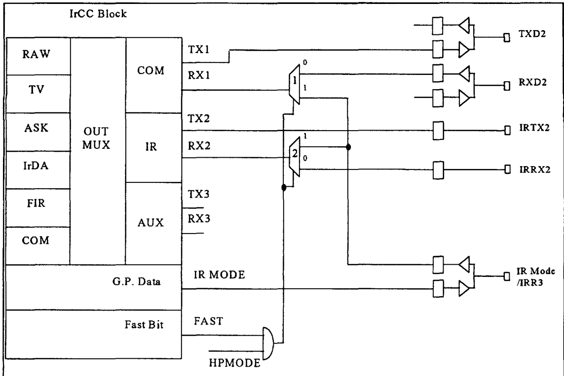
Figure F1 - Fast IR Interface Block Diagram
